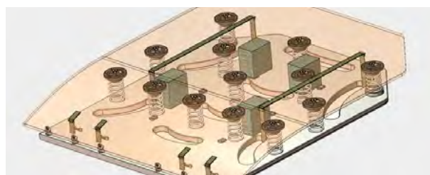
13 muelles dinámicos específicamente adaptados al salto
